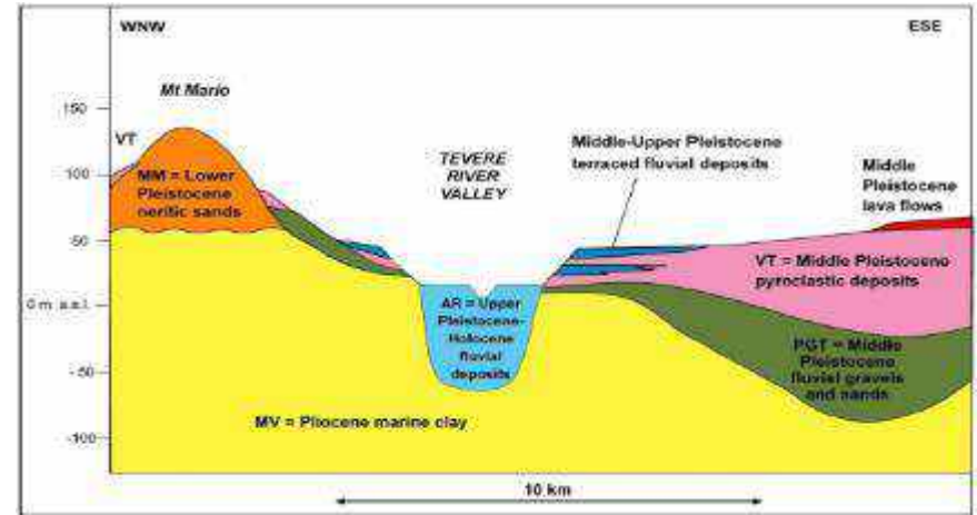
Schema dei rapporti stratigrafici nell'area urbana di Roma.
